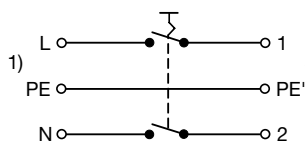
Netzschalter unbeleuchtet
