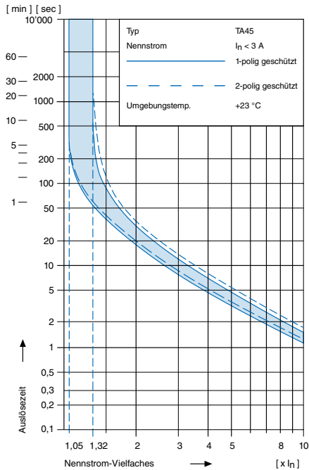
Auslösekennlinien I_n < 3\text{ A}
