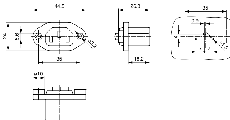
Montageflansch mit Durchgangslöchern Sonderausführung
