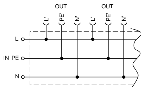
Verteilleiste mit 5 Gerätesteckdosen und Wippenschalter beleuchtet
