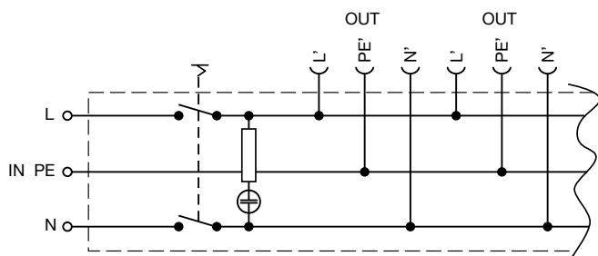
Verteilleiste mit 5 Gerätesteckdosen und Wippenschalter beleuchtet
